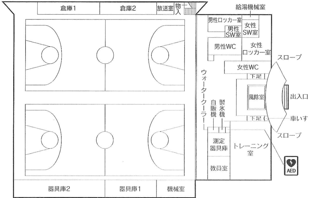
【1階平面図】
