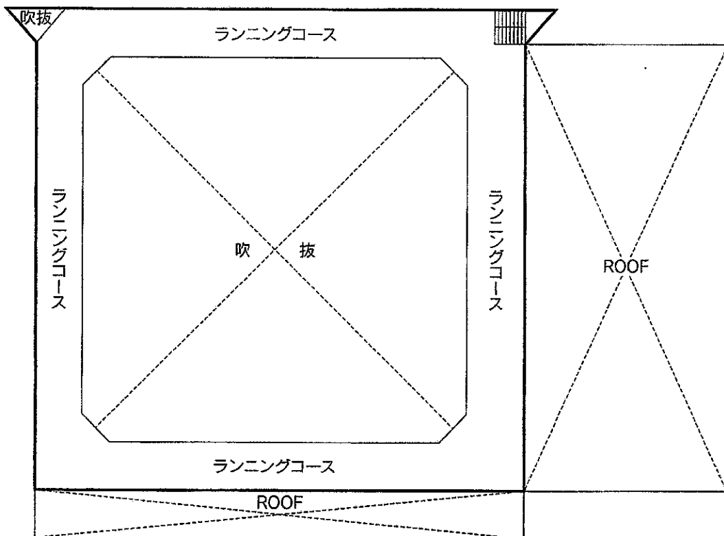
【2階平面図】
